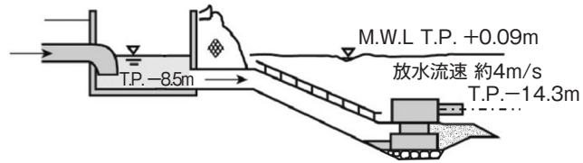
放水管式水中放水方式 (玄海原子力発電所3,4号機)
